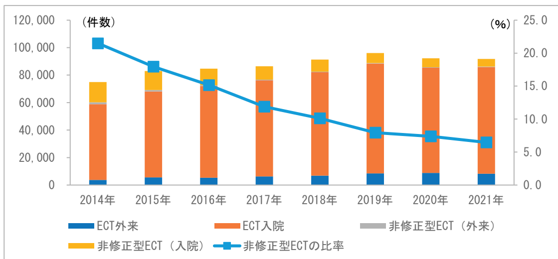
図2 ECT件数の推移（全国）
