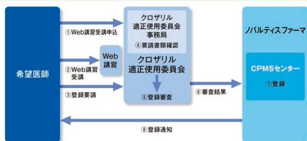
図2 CPMS運用手順 改訂 6.2版 P24
